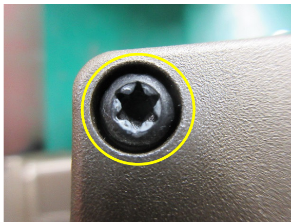
変更後：ヘックスローブ（トルクス） 規格：T25
